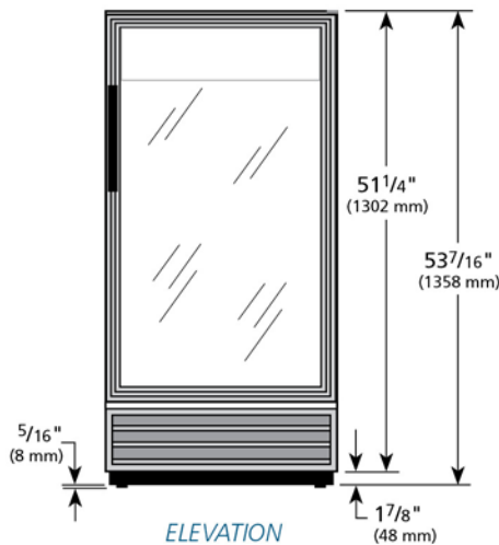
ELEVATION
